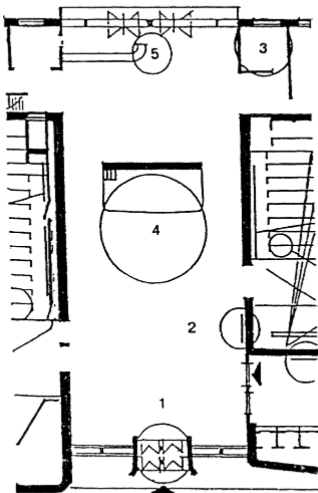
Пример приспособления фойе типового кинотеатра (N 264-13-101) к посещению инвалидами
