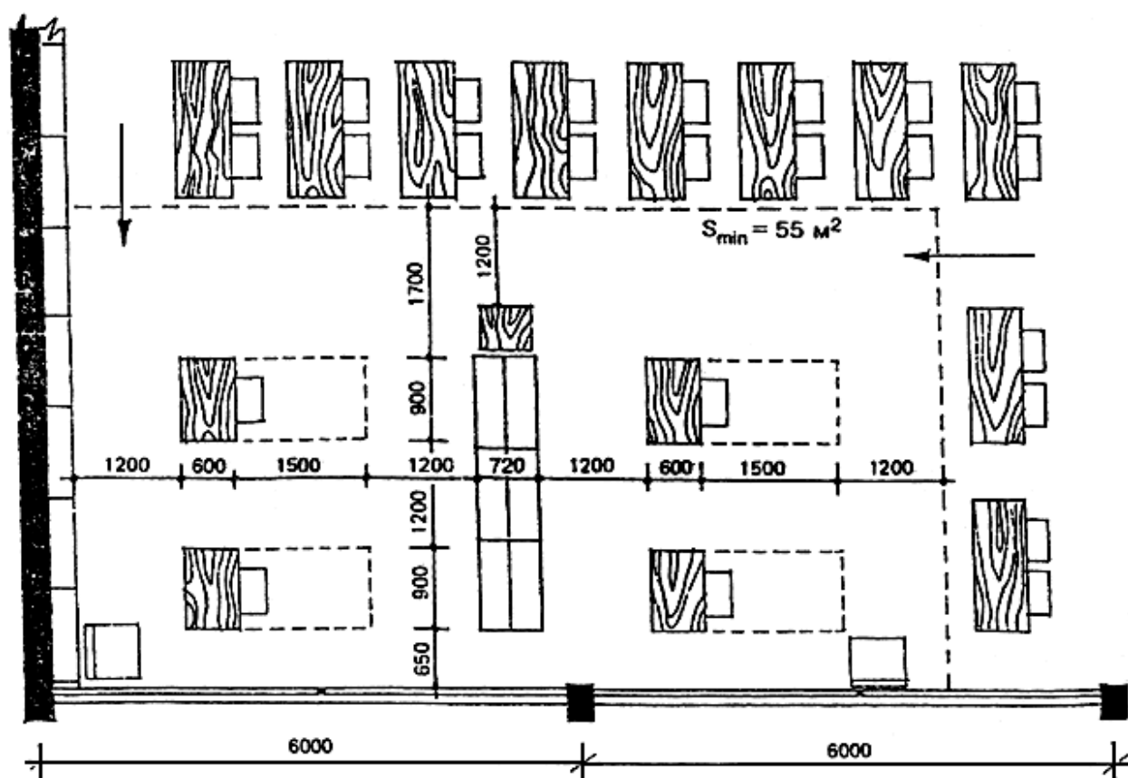
Специализированное читальное отделение в городской библиотеке
