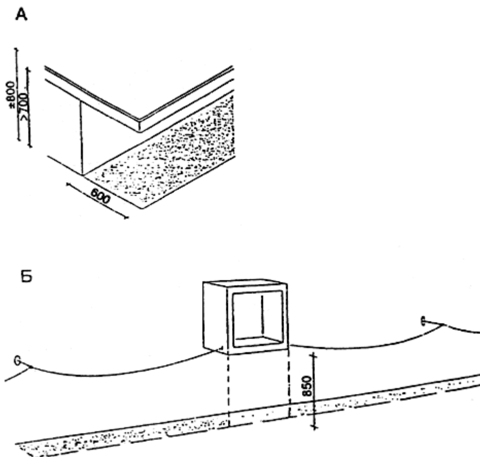
Варианты и основные параметры демонстрационных витрин для инвалидов на колясках
