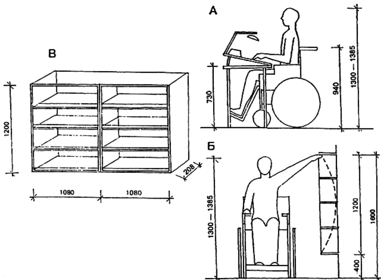
Библиотечное оборудование для инвалидов
