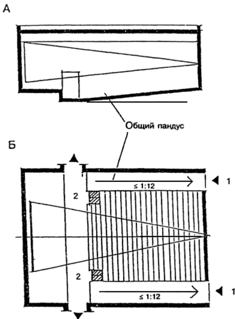
Пример решения загрузки и эвакуации инвалидов-колясочников в кинозалах с уклоном пандусов менее 1:12
