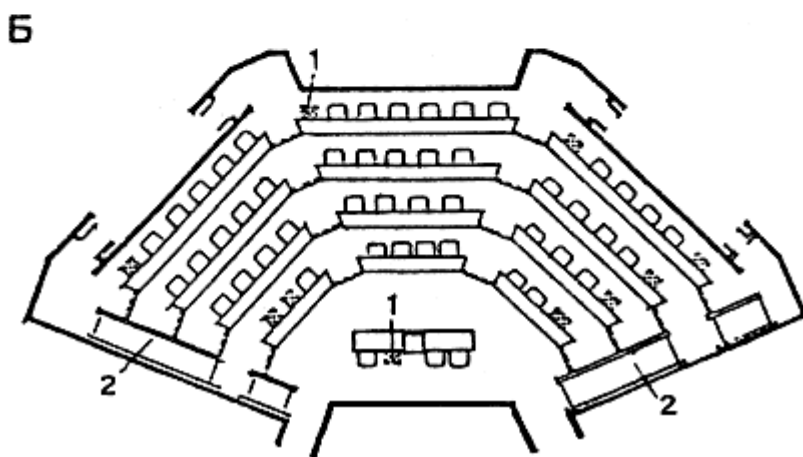
Возможные формы лекционных залов и рекомендуемые места размещения инвалидов-колясочников
