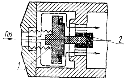
1 — пружина сжатия; 2 — плавкий элемент (например расплавляющийся припой)
