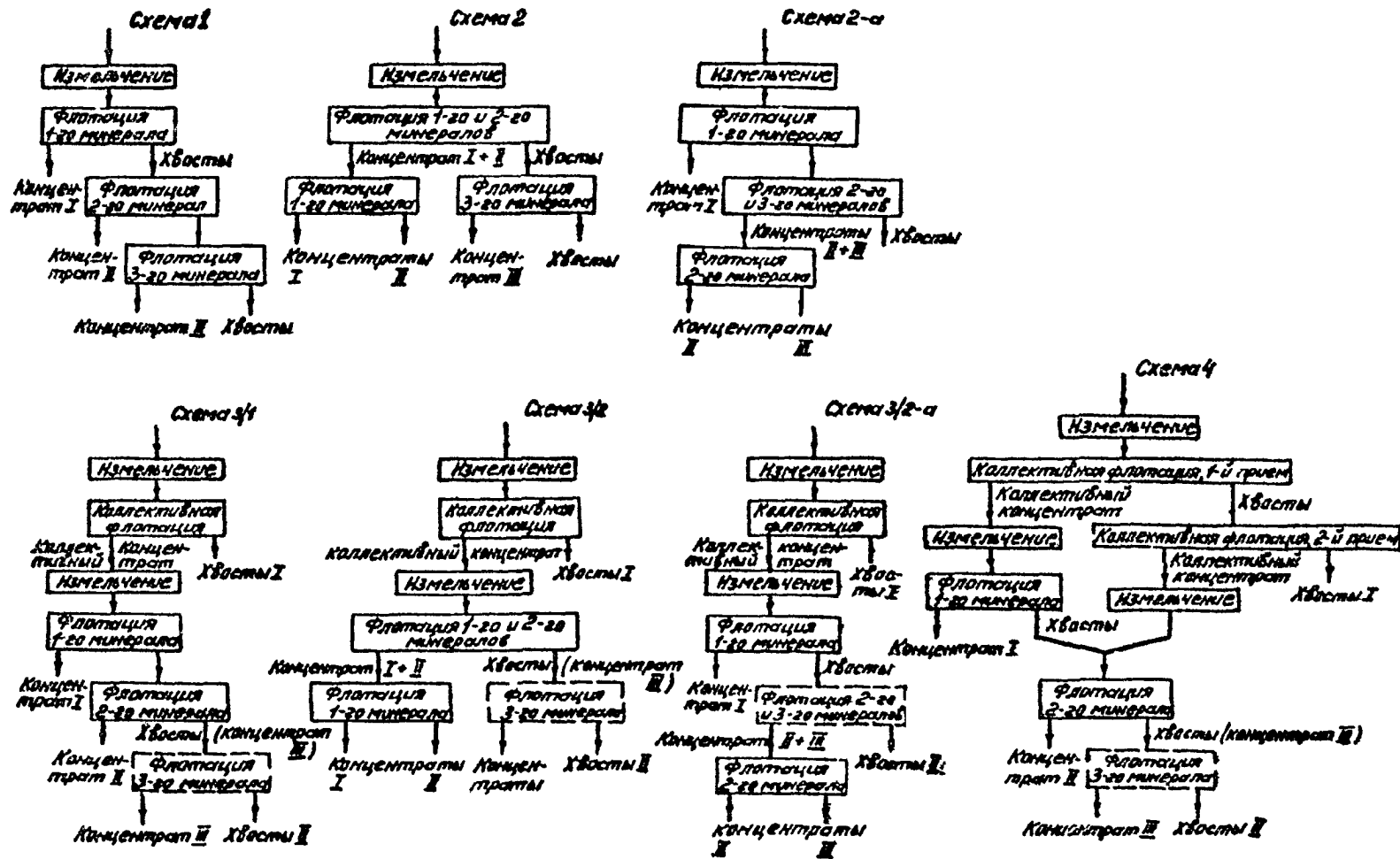
Рис. 7 Принципиальные схемы флотации полиметаллических руд содержащих при палезных компонентах
