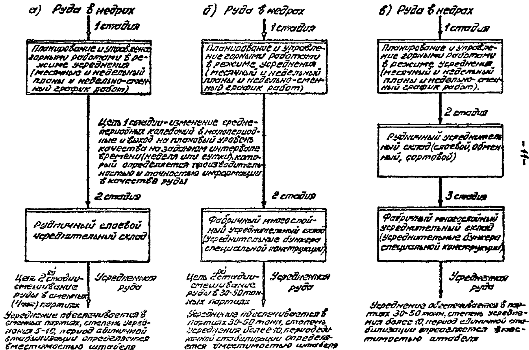
Рис. 2 Принципиальные схемы усреднения руды для валового усреднения
