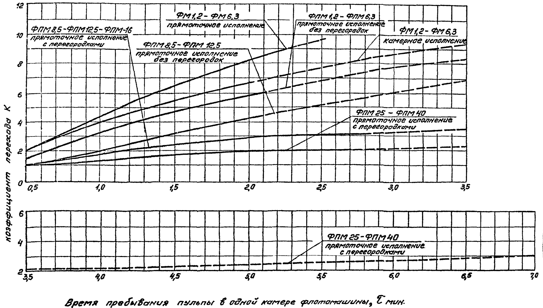
Рис. 8 Зависимость K от \tau для флотационных машин различных типов
