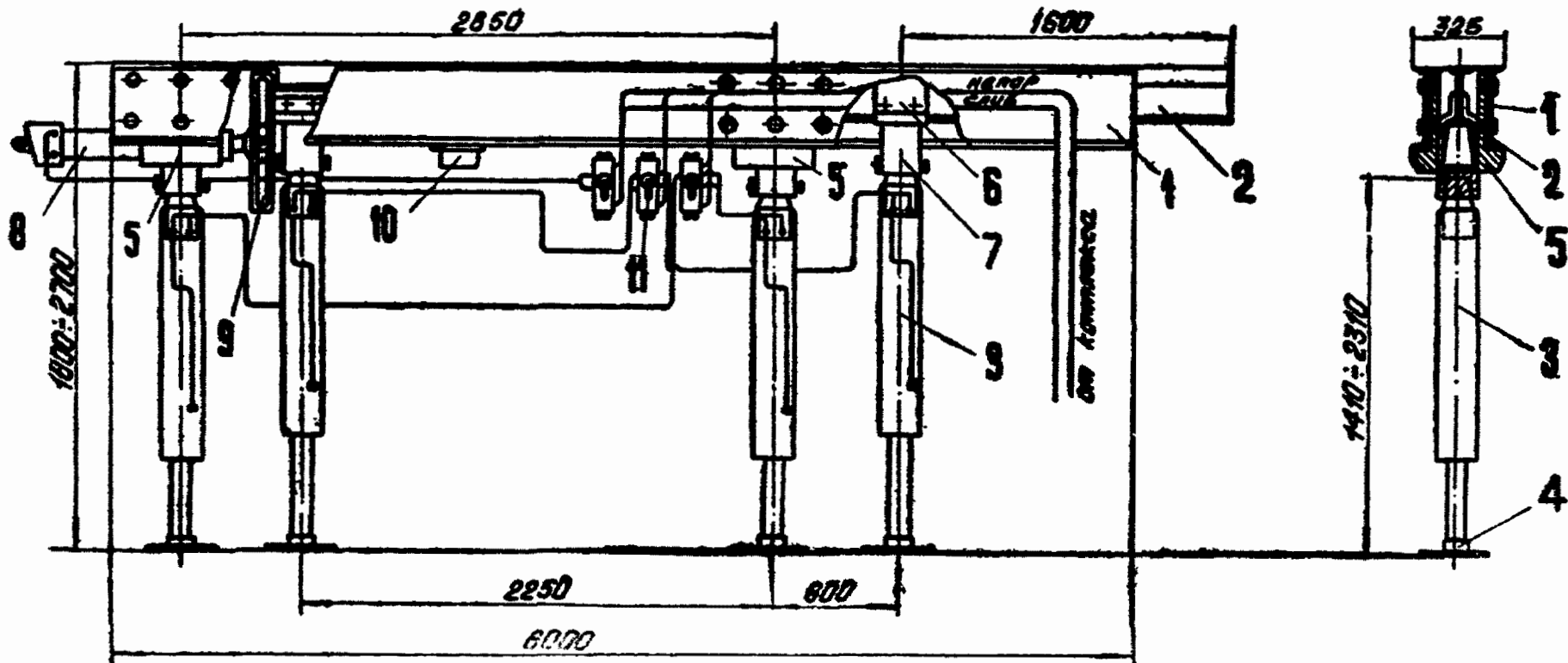
Рис. 3.3. Гидрофицированная крепь сопряжения конструкции шахты «Зыряновская».
