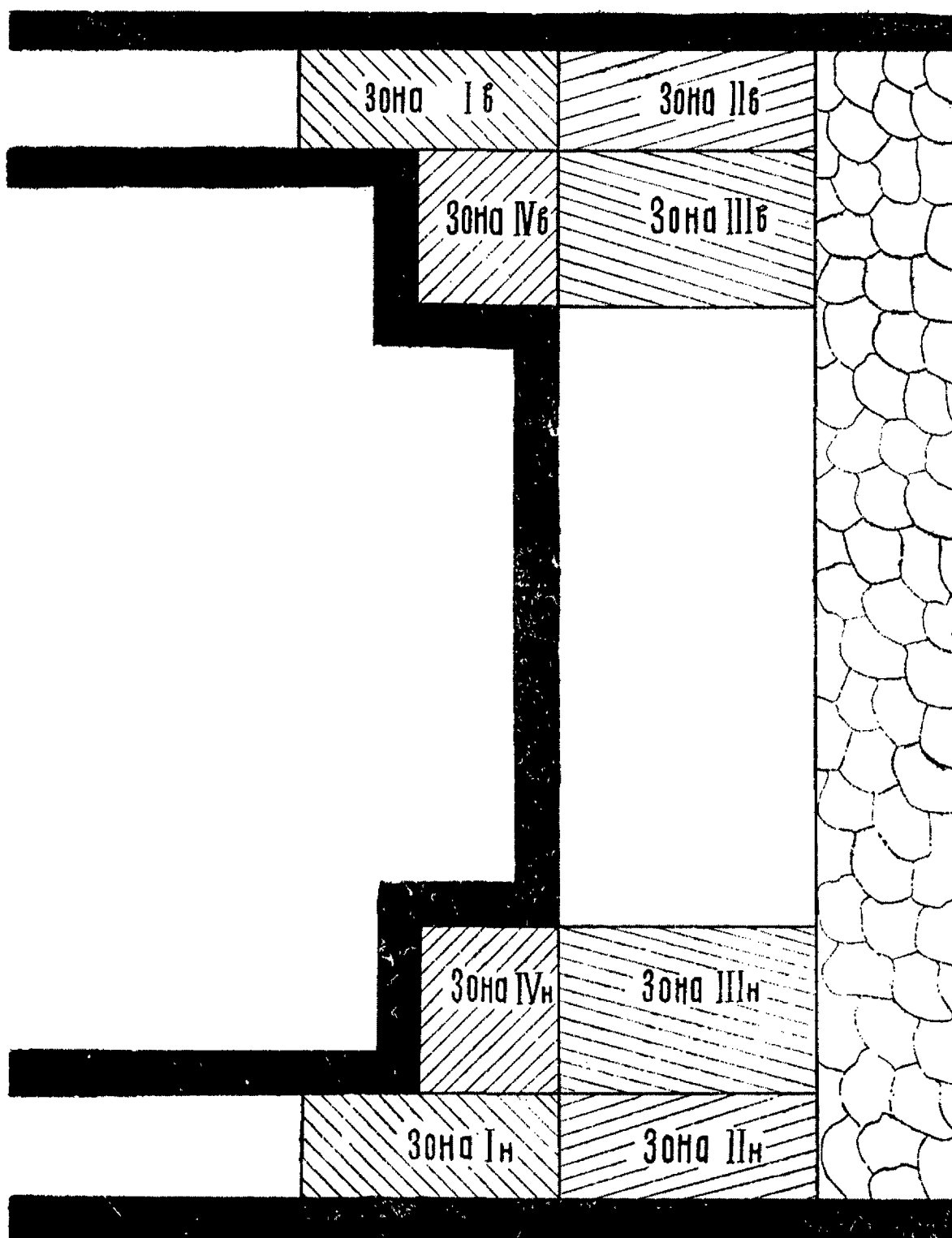
Рис. 1.1. Рабочие зоны сопряжений лав со штреками.
