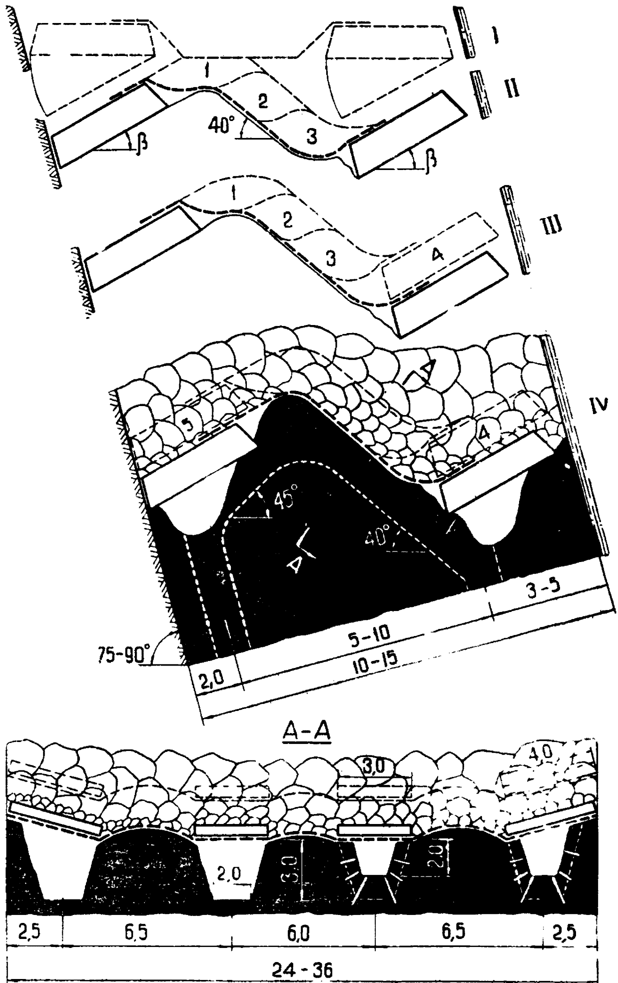
Рис. 8. Управление перекрытием в односкатном забое с наклоном к кровле пласта при выемке угля в межщитовом целике полосами по простираанию в нисходящем порядке
