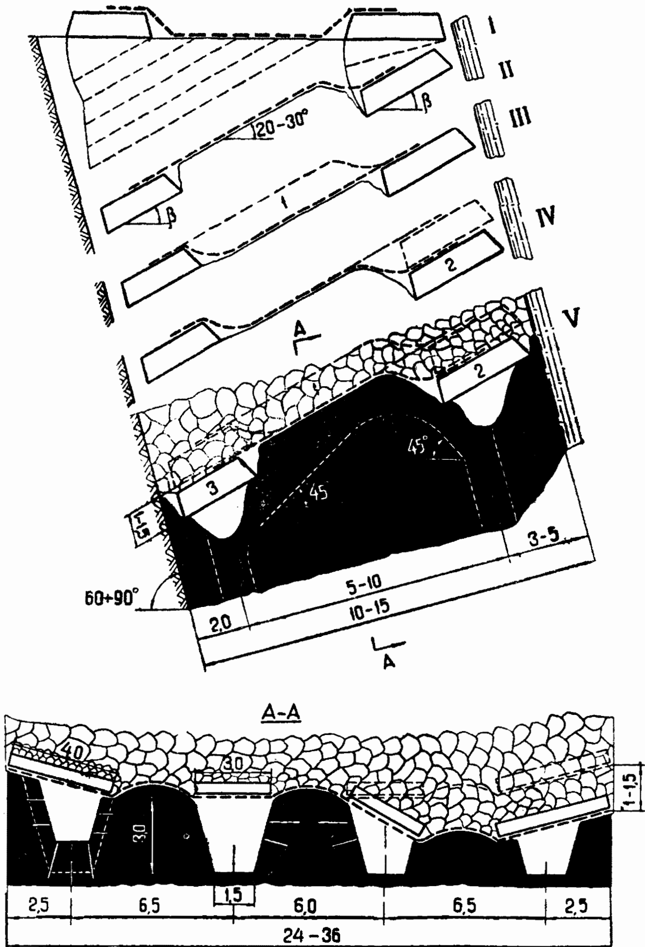
Рис. 5. Управление перекрытием в односкатном забое с наклоном к почве пласта при выемке угля в межщитовой толще полосами вкрест простираения пласта
