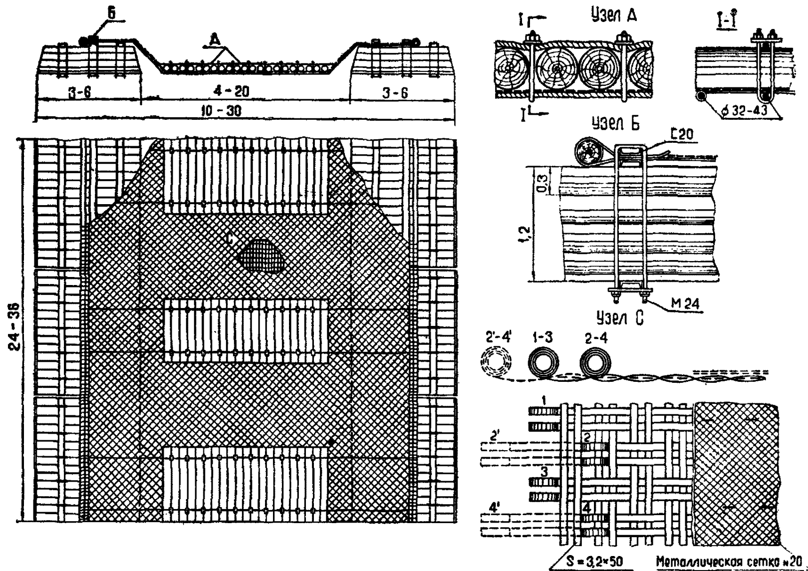
Рис. 3. Конструкция комбинированного перекрытия УКГП: А — крепление ребер жесткости на гибком перекрытии; Б — крепление гибкого перекрытия к щитам; С — схема переплета металлических лент основы гибкого перекрытия
