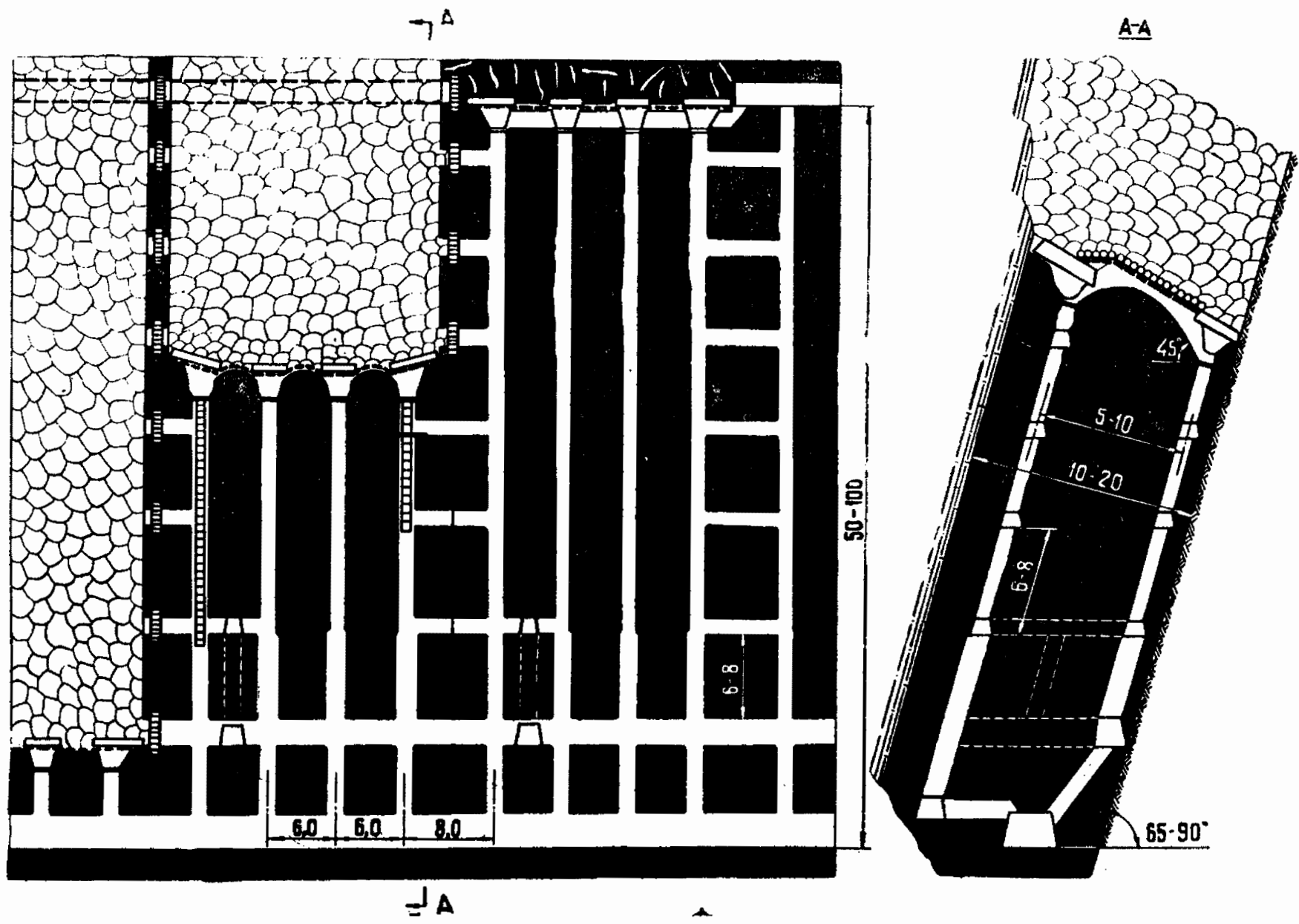
Рис. 1. Система разработки мощных крутых пластов столбами по падению с применением комбинированных перекрытий УКПП
