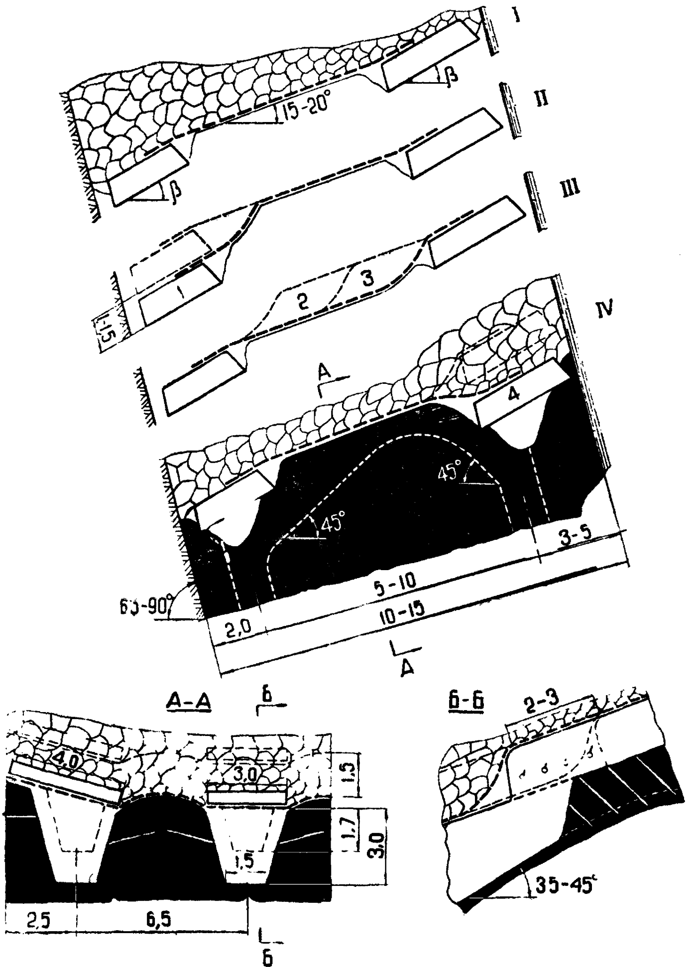
Рис. 7. Управление перекрытием в односкатном забое с наклоном к почве пласта при выемке угля в межщитовой толще полосами по простиранию в восходящем порядке
