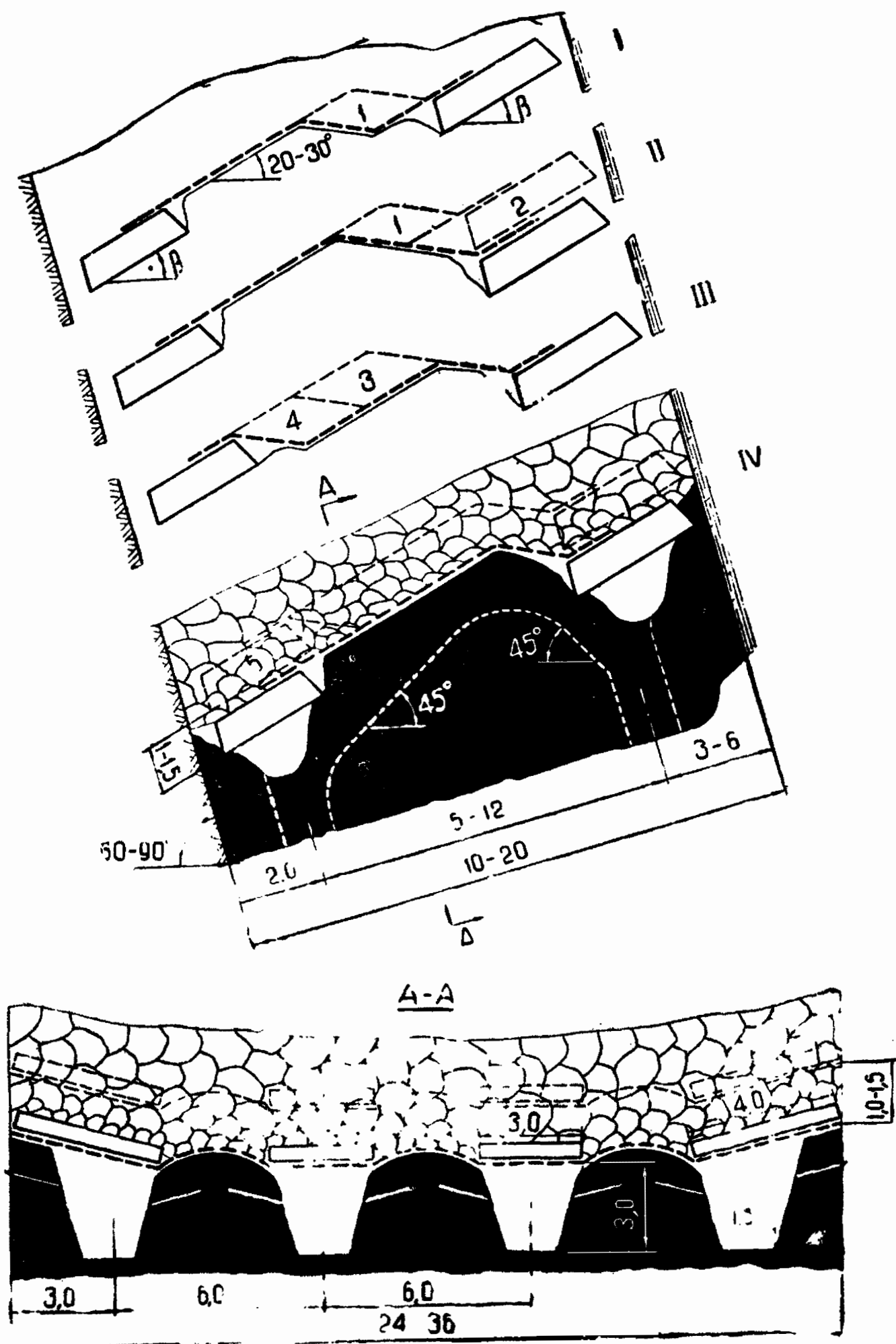
Рис. 6. Управление перекрытием в односкатном забое с наклоном к почве пласта при выемке угля в межщитовой толще полосами по простиранью в нисходящем порядке
