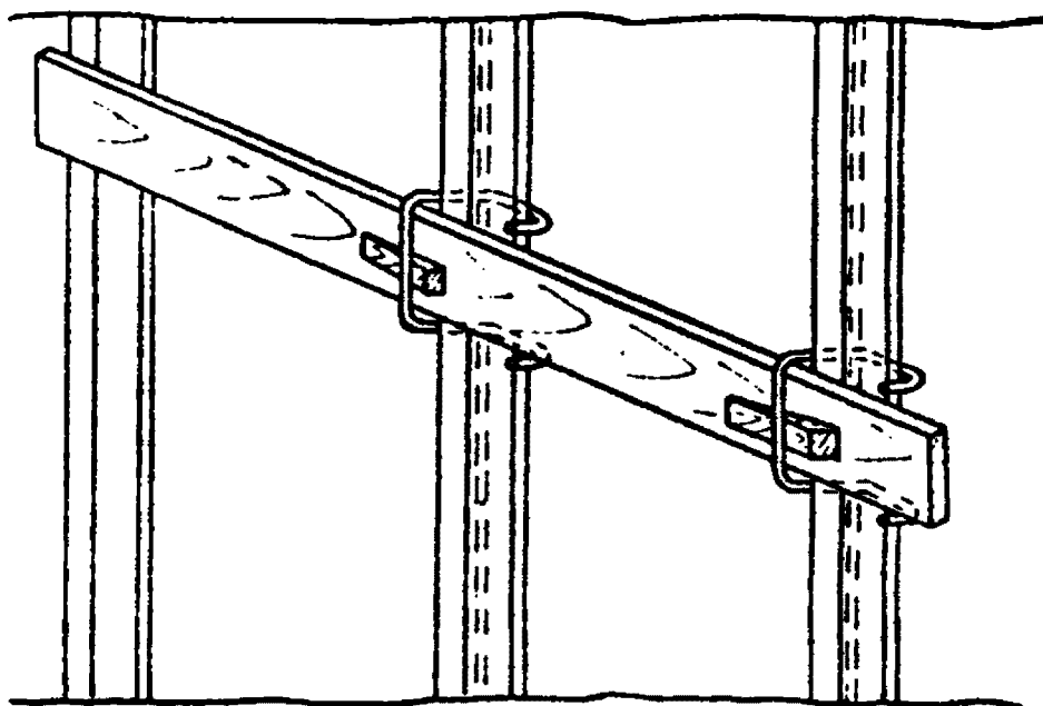
Рис. 4. Шаблон для установки рамы
