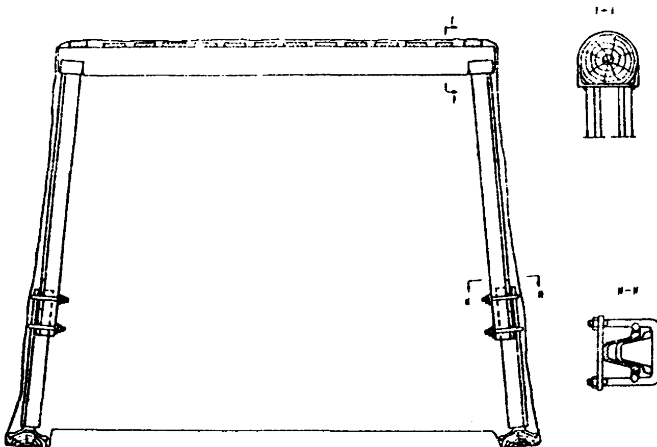
Рис. 3. Металлическая трапециевидная податливая крепь с деревянным верхняком (МТД)
