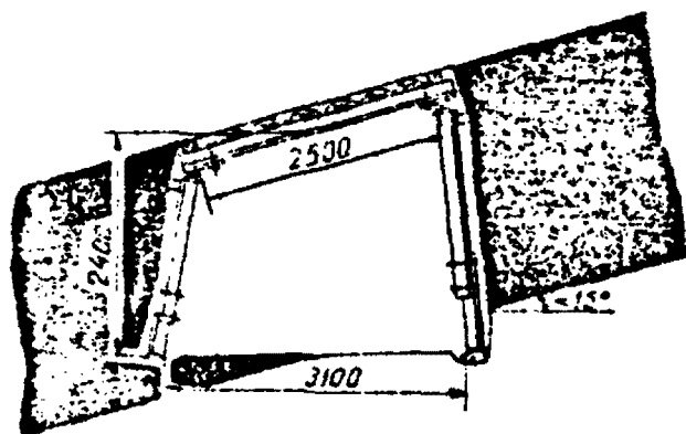
Поперечный разрез
