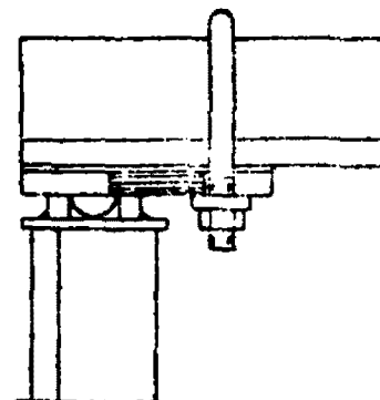
Детали крепл.
