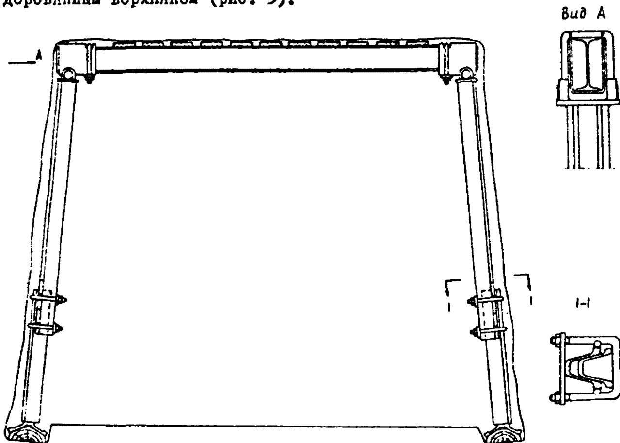
Рис. 2. Металлическая трапецевидная податливая крепь с двутавровым верхняком (МТПА)
