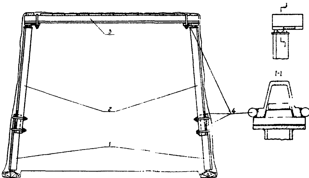
Рис. 1. Металлическая трапецевидная податливая шарнирная крепь (МТПШ)
